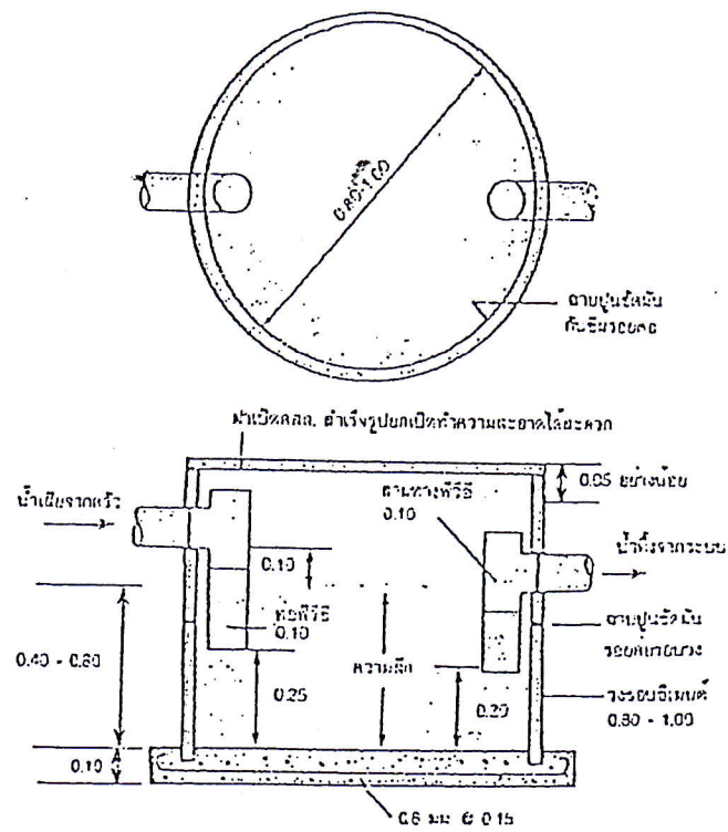
บ่อดักไขมันแบบวงขอบซีเมนต์สำหรับพักอาศัย
